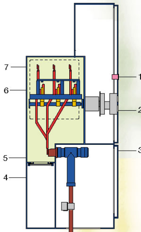
Ячейка выключателя нагрузки
