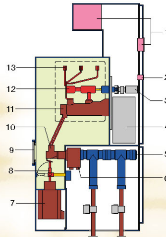
Ячейка силового выключателя на 1250 А
