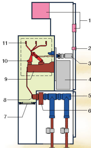
Ячейка силового выключателя на 630 А
